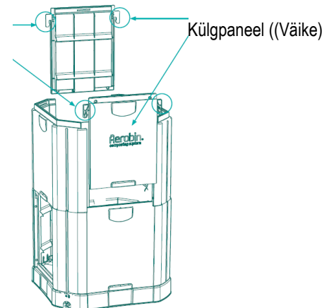
Külgpaneelide konksud
